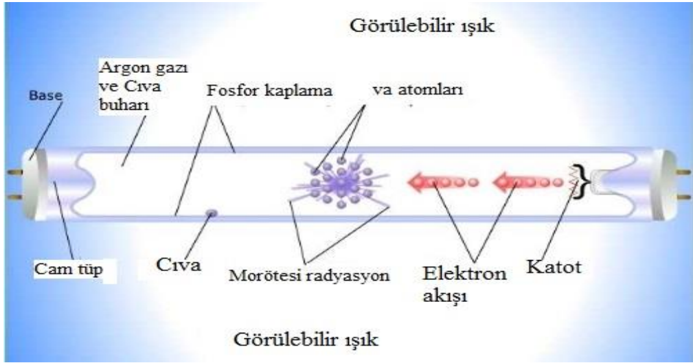
Şekil 1.1.4.1. Floresan Lamba Yapısı (Anonim, 2017)
