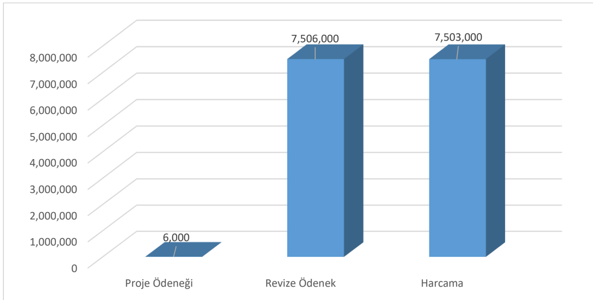
Şekil 9: İhtisaslaşma Projesi
